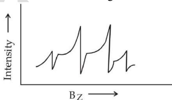
Fig. 6.12. ESR spectrum of \dot{\text{C}}\text{H}_3
